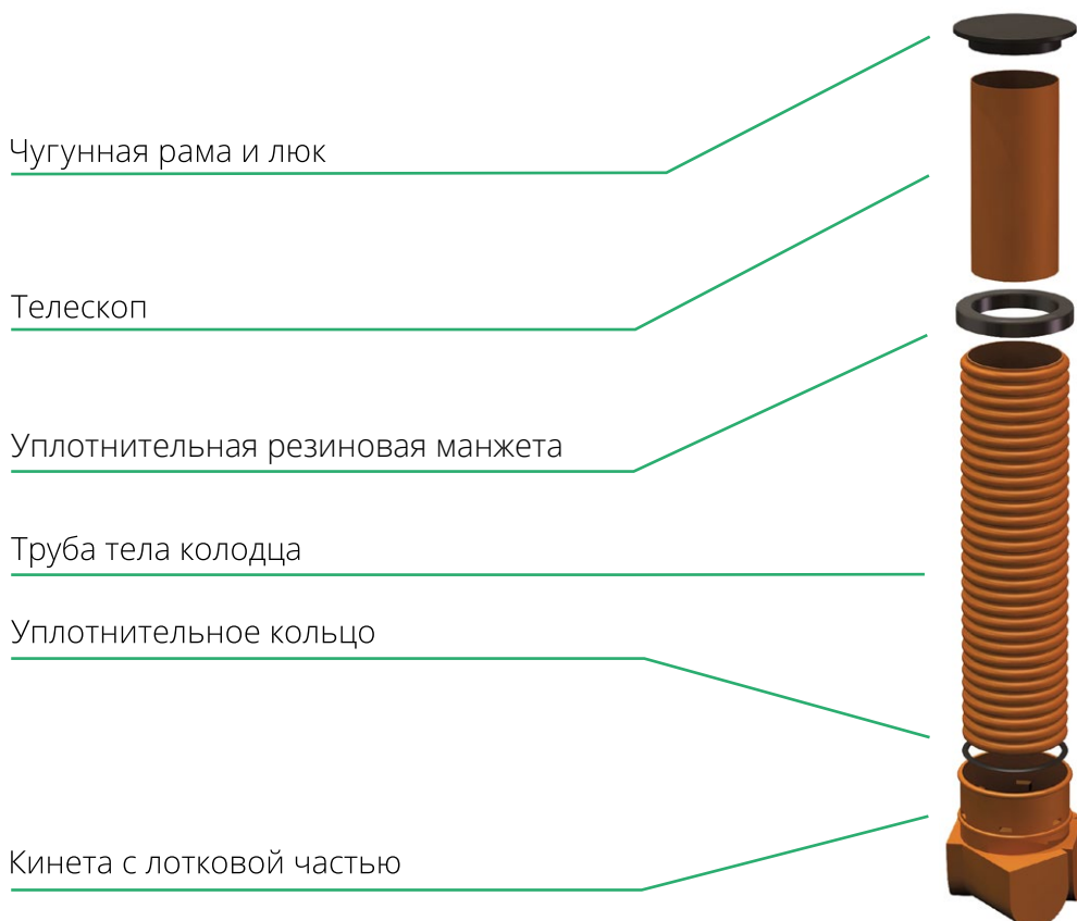
Рисунок: Модульная конструкция колодца Nawell Ø400
