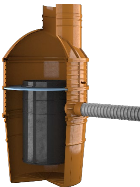
Рисунок: Фильтр патрон
