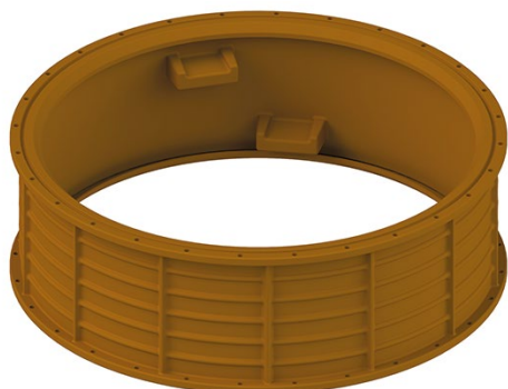
Рисунок: Тело колодца: Н=500мм
