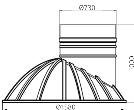
Рисунок: Конус-переход для колодца Nawell Ø1500
